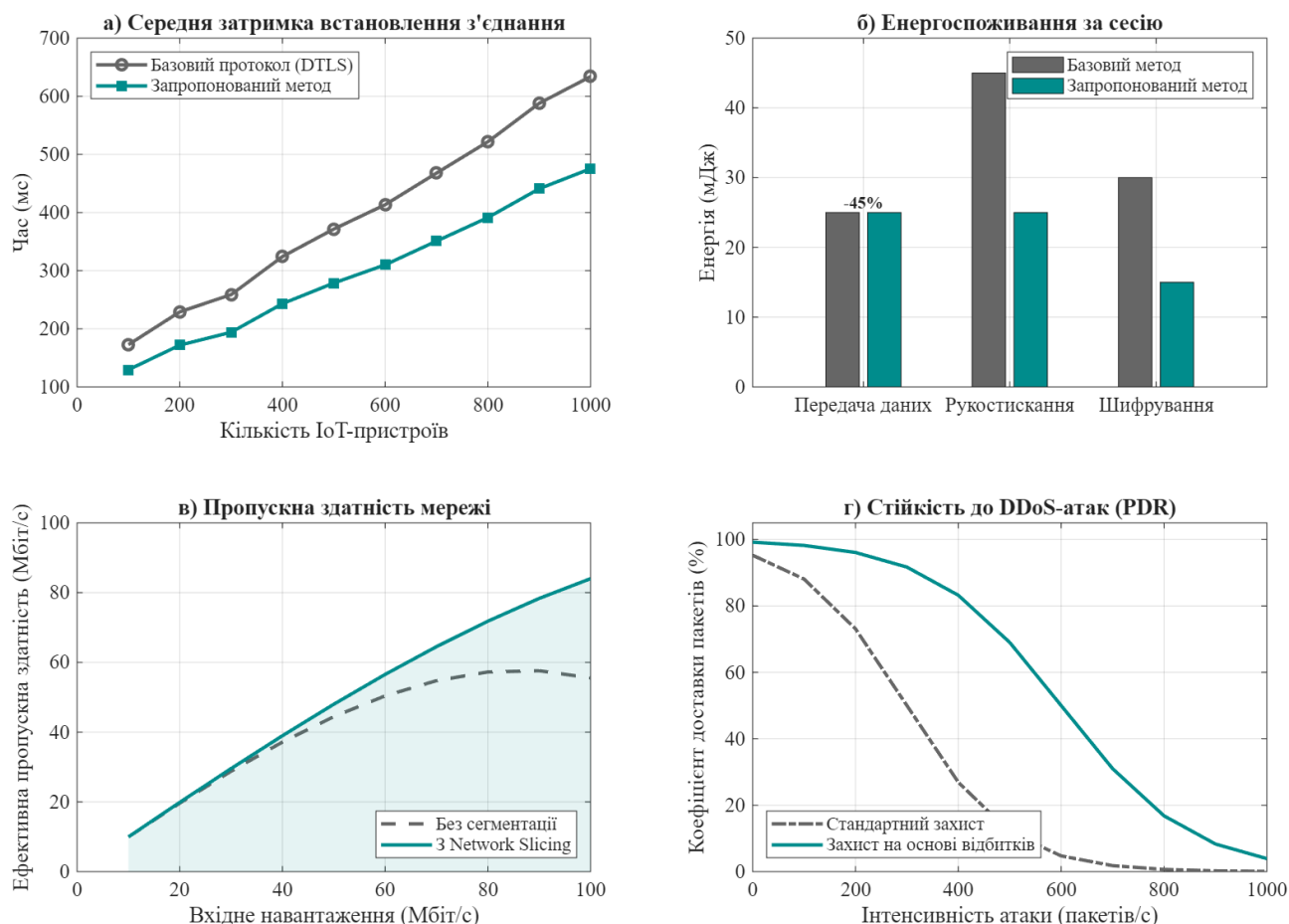
Рис. 4. Результати порівняльного аналізу ефективності розробленого методу захисту (AES-128/ECC + Device Fingerprinting) та базового протоколу (DTLS + RSA + X.509): а) залежність середньої затримки автентифікації від кількості пристроїв; б) порівняння енергоспоживання на етапах встановлення з'єднання; в) динаміка пропускної здатності каналу при збільшенні навантаження; г) стійкість до втрат пакетів (PDR) в умовах DDoS-атаки
