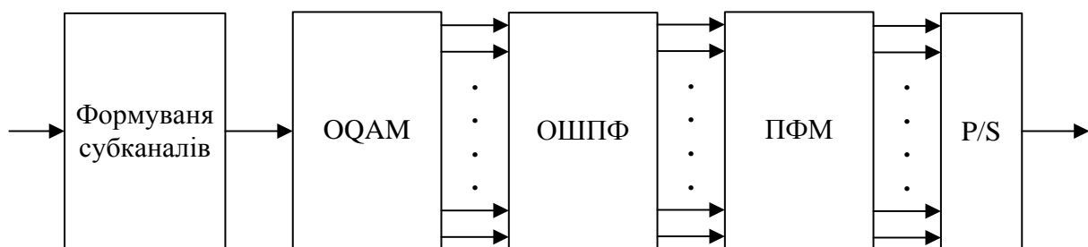
Рис. 1. Блок-схема FBMC-модуляції
