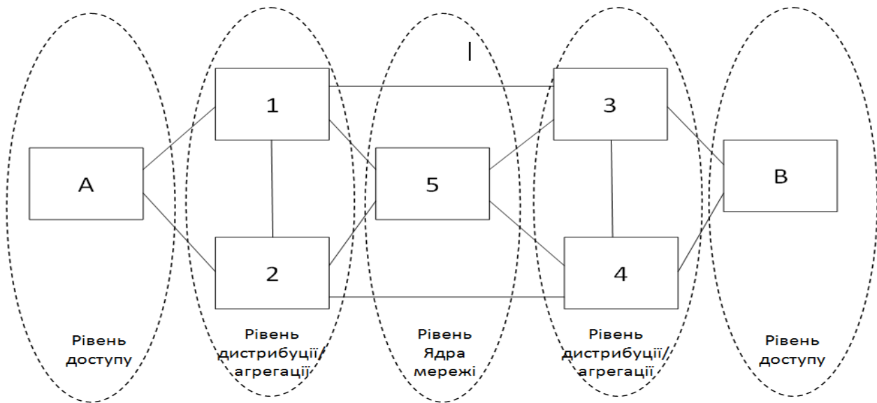
Рис. 2. Топологія сучасної телекомунікаційної мережі
