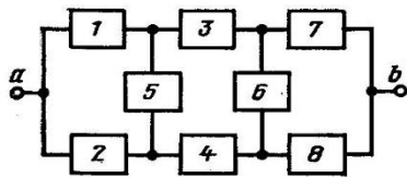
Рис. 4. Подвійна місткова схема з'єднання елементів
