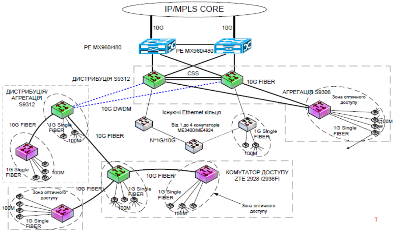
Рис. 1. Узагальнена архітектура телекомунікаційної мережі майбутнього
