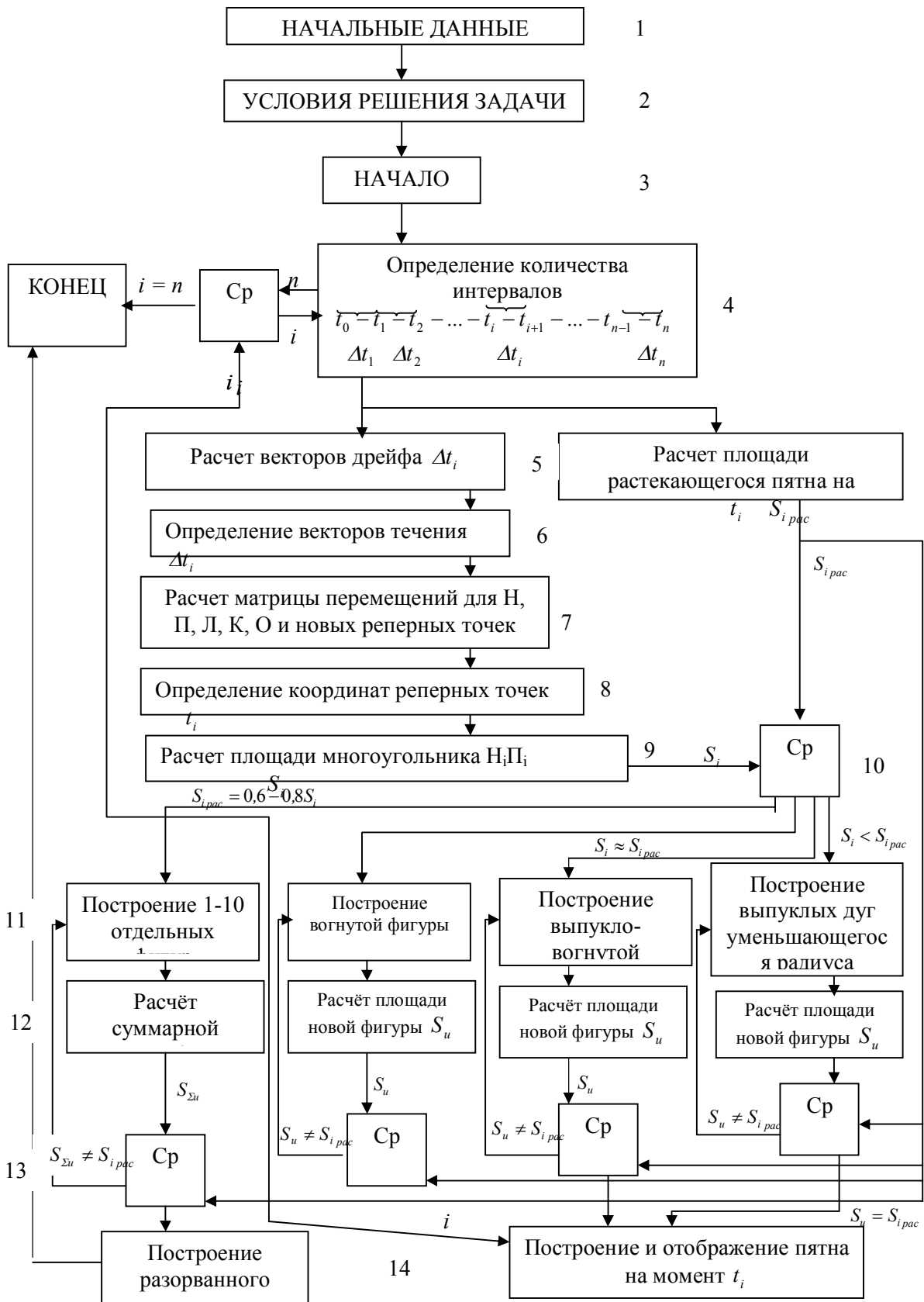
Рис.1. Структурная схема алгоритма управления экологической безопасностью.
