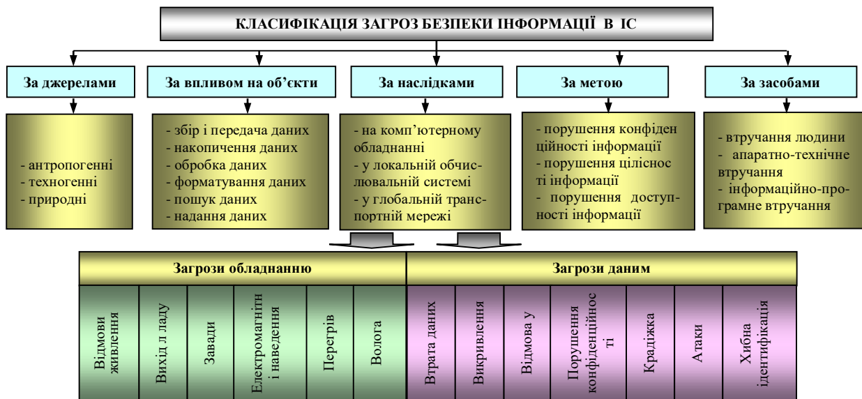
Рис. 1. Загальна класифікація комп'ютерно-телекомунікаційних загроз
