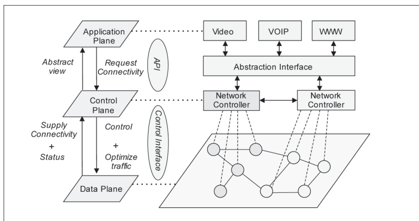
Рис. 2. Концепція SDN
