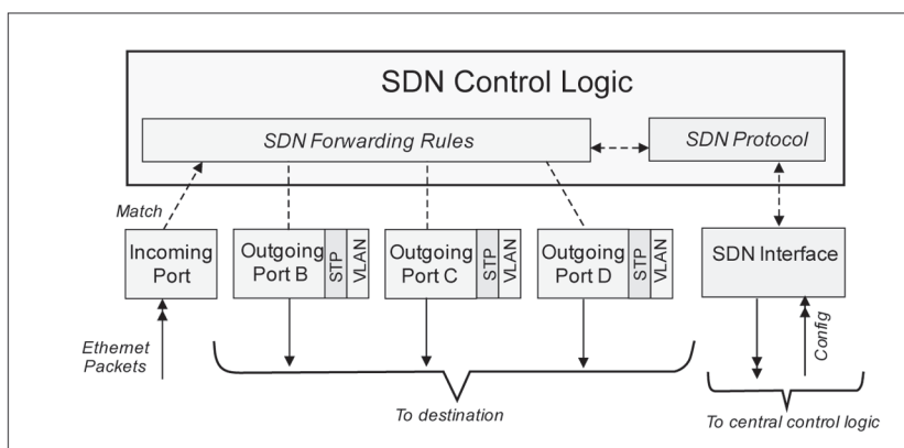
Рис. 3. Комутатор SDN
